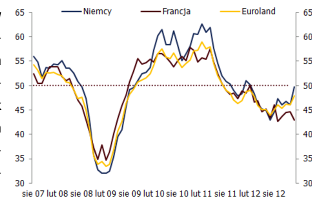
Rys. 4. Indeksy PMI
